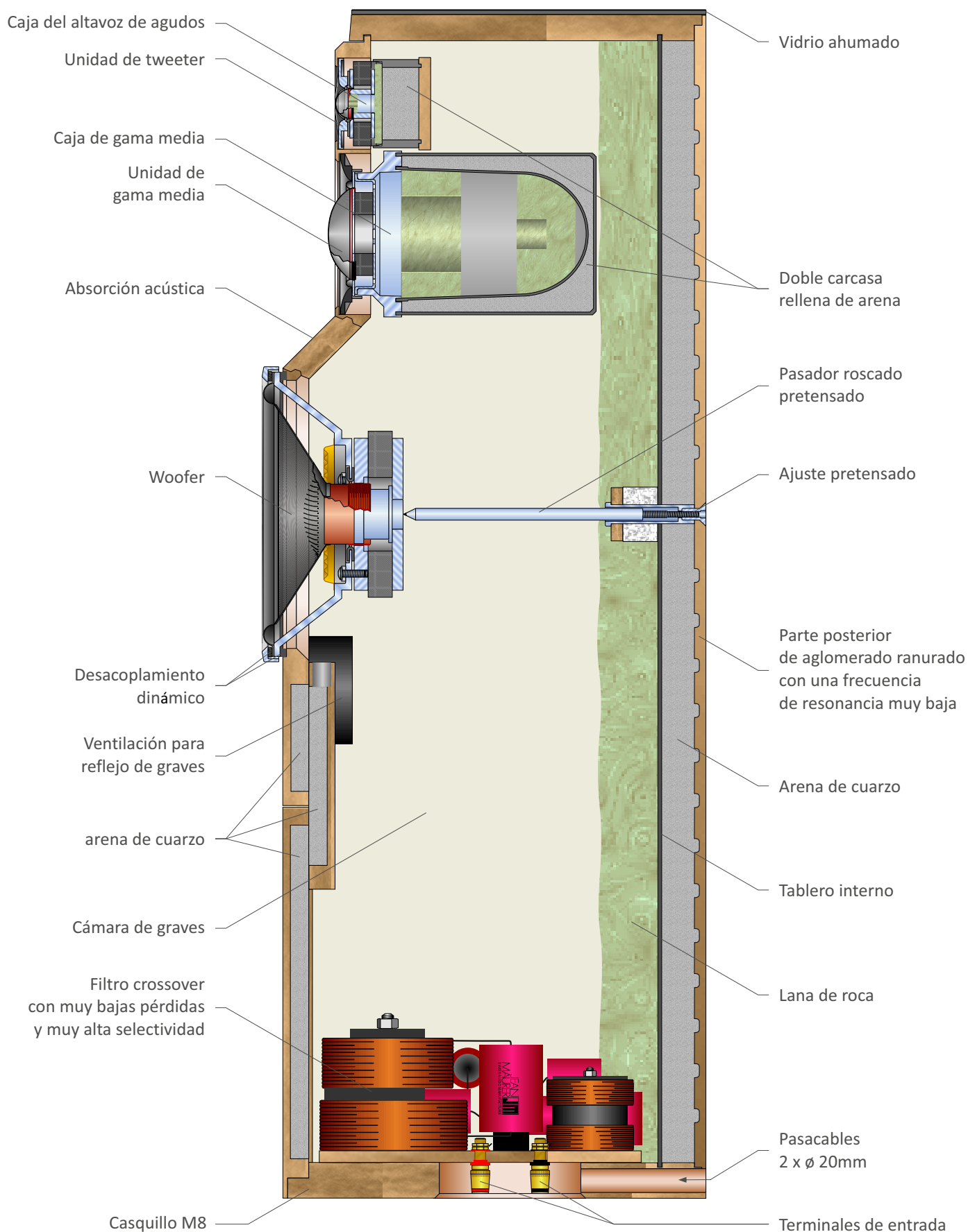
Vista en corte de la caja acústica JM 370F
