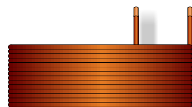
Bobinado de autoinducción sin núcleo y con una sección transversal muy grande: 1,68 mH - 0,11 \Omega - 3 kg
