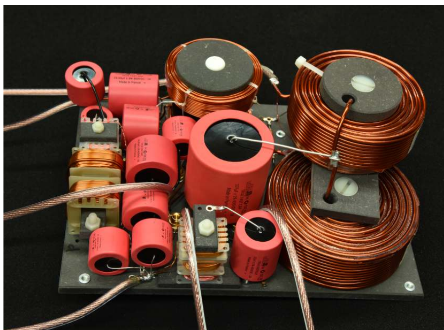
Bobinado de autoinducción sin núcleo y con una sección transversal muy grande: 1,68 mH - 0,11 \Omega - 3 kg
