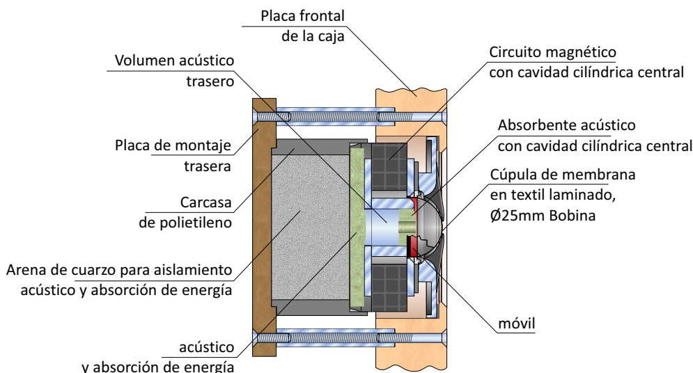
Caja de agudos, con transductor TD25-4
