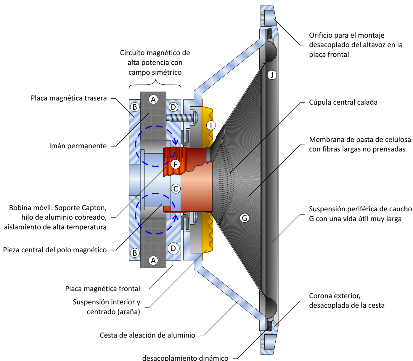
B245-5 woofer
