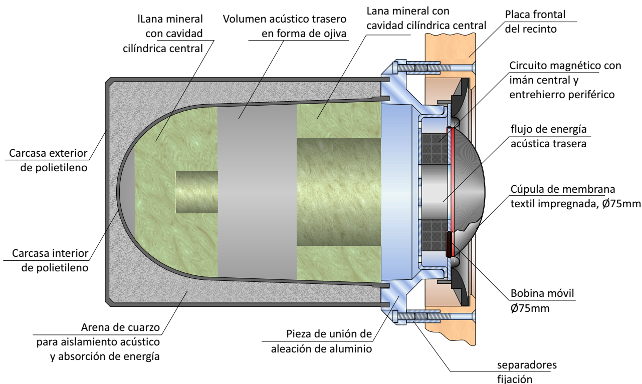
Recinto de rango medio, con transductor MD75-3
